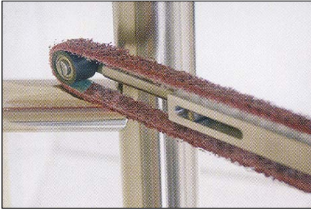
ROHR-FIX VAIHTOPÄÄLLÄ PUTKIJUUREN SATINIHIONTAA KARHUNKIELINAUHALLA.
