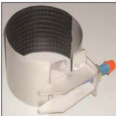
TF10 1-OSAINEN PANTA PAINE: 16 BAR ALUE: 20-276 mm PITUUS: 75, 150 mm
