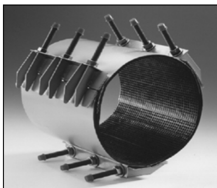
TS30 3-OSAINEN PANTA PAINE: 10/6/4/2 BAR ALUE: 270-1000 mm PITUUS: 300, 400, 500, 600, 700mm
