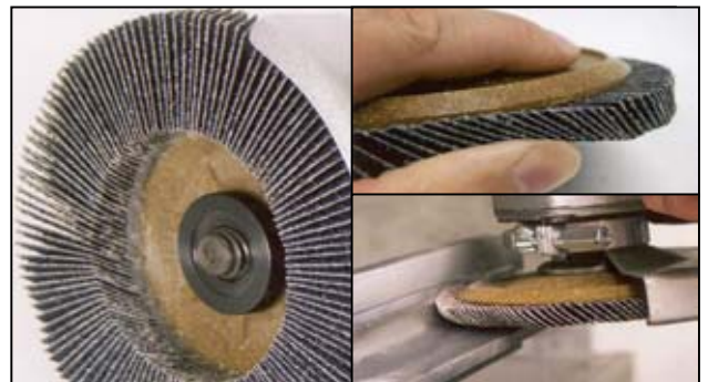
PLANTEX TRIMTEX LIUSKAKIEKKO KASVIMASSARUNGOLLA SAKSASTA MONIKÄYTTÖKIEKKO SUURELLA MÄÄRÄLLÄ LIUSKOJA. "PEHMEÄ-JOUSTO-AJO". 63 m/s. KULMIIN / HITSISAUMAT. MAKS 9700 RPM
